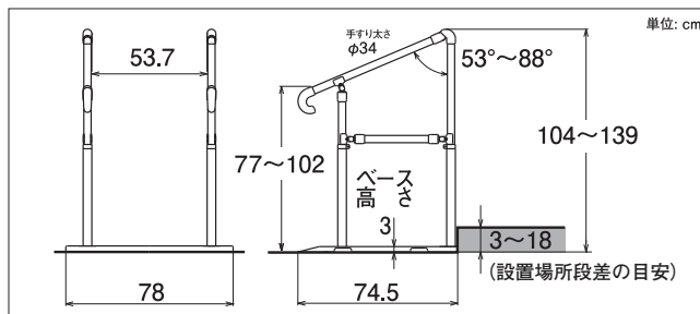
CKH-01 ステップ台 1段仕様
