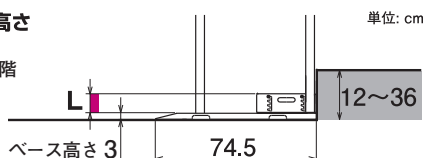
両手すり(CKH-01) +ステップ台 1段
