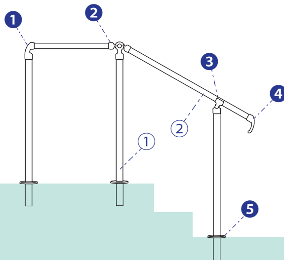
手すり形状：丸パイプ
