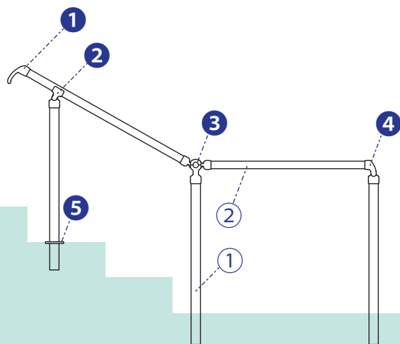
手すり形状：丸パイプ
