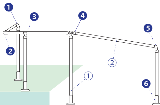
手すり形状：丸パイプ
